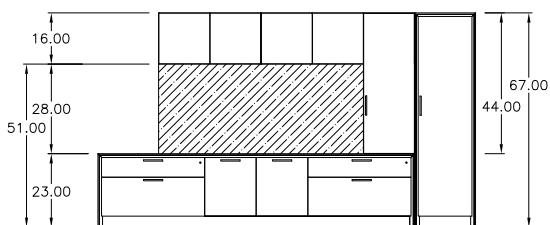
Elevation 2
