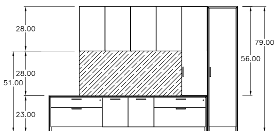
Elevation 3
