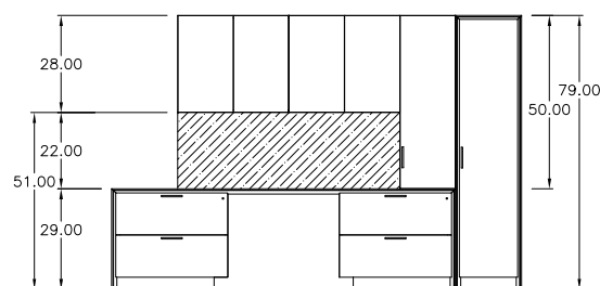
Elevation 5
